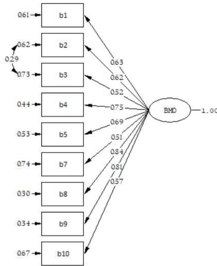
Şekil 1. Birinci düzey DFA'ya ilişkin Path diyagramı.
